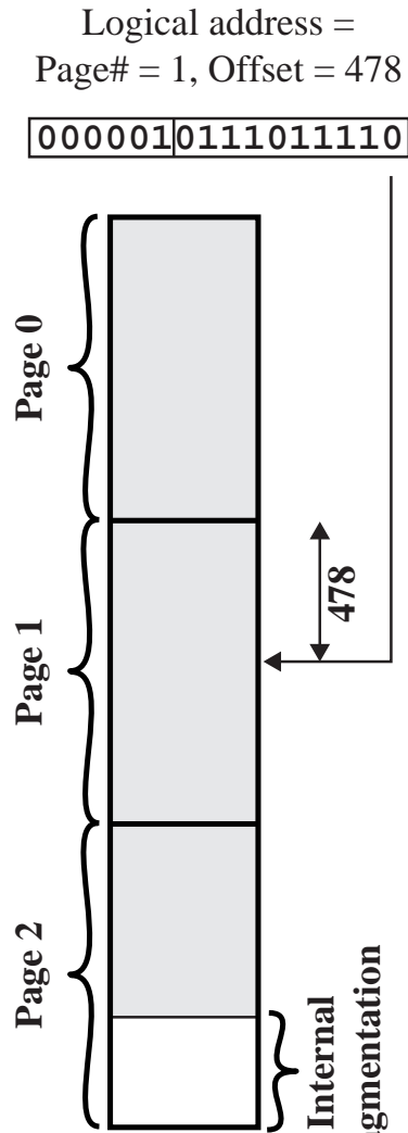
(b) Paging (page size = 1K)
